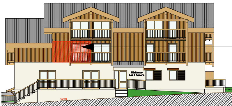
FACADE OUEST
