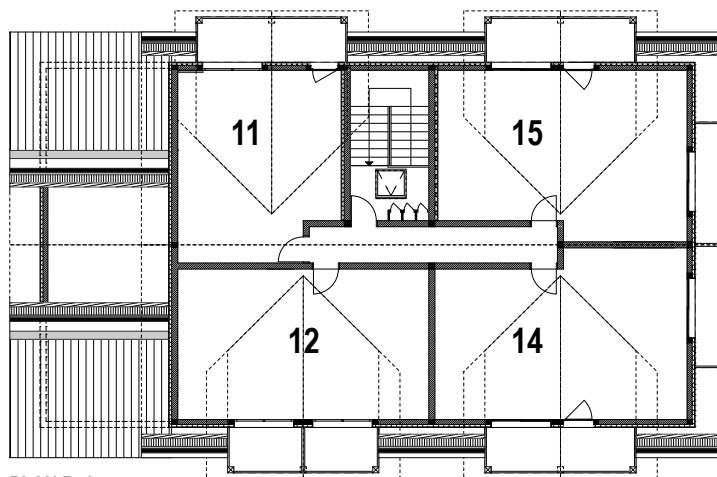
PLAN R+2
